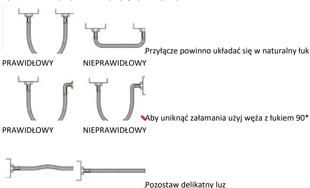
Rys.1 Zalecenia przy montażu przyłączy elastycznych:
